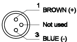
2 wire QD wiring
