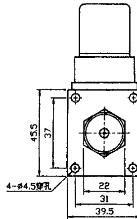
壓力接頭外部尺寸圖
