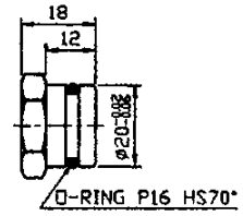
壓力接頭外部尺寸圖
